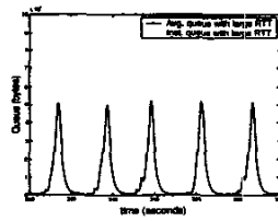
Fig. 15. 45 ECN FTP (large RTT)
