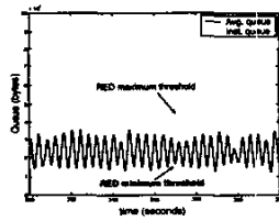
Fig. 7. Queue - 15 ECN FTP
